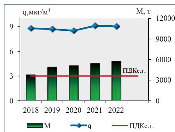
Рис. 3.14. Среднегодовые концентрации формальдегида ( q , \mu\text{г}/\text{м}^3 ) и выбросы от стационарных источников ( M , т)
