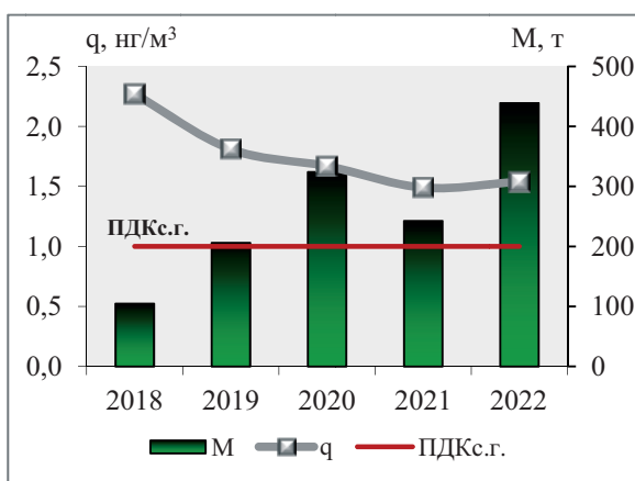
Рис. 3.13. Среднегодовые концентрации бенз(а)пирена ( q , \text{нг}/\text{м}^3 ) и выбросы от стационарных источников ( M , т)
