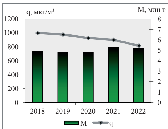
Рис. 3.11. Среднегодовые концентрации ( q , \mu\text{г}/\text{м}^3 ) и выбросы от стационарных источников ( M , млн т) оксида углерода
