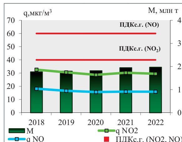
Рис. 3.12. Среднегодовые концентрации диоксида азота ( q\text{NO}_2 , \mu\text{г}/\text{м}^3 ) и оксида азота ( q\text{NO} , \mu\text{г}/\text{м}^3 ) и выбросы от стационарных источников ( M , млн т) \text{NO}_x (в пересчете на \text{NO}_2 )
