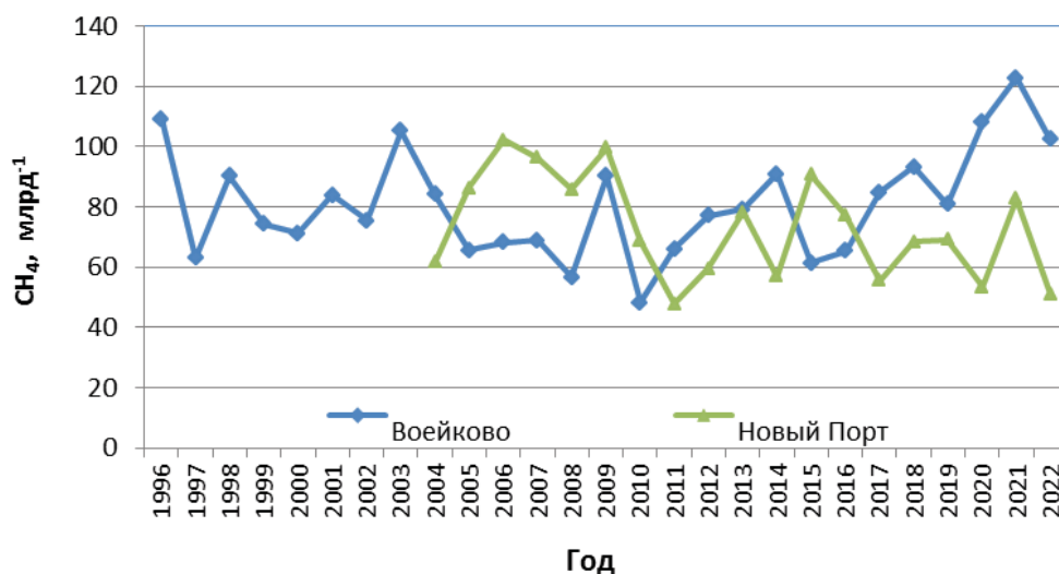
Рис. 2.3. Среднегодовое превышение концентрации CH 4 над фоновым уровнем
