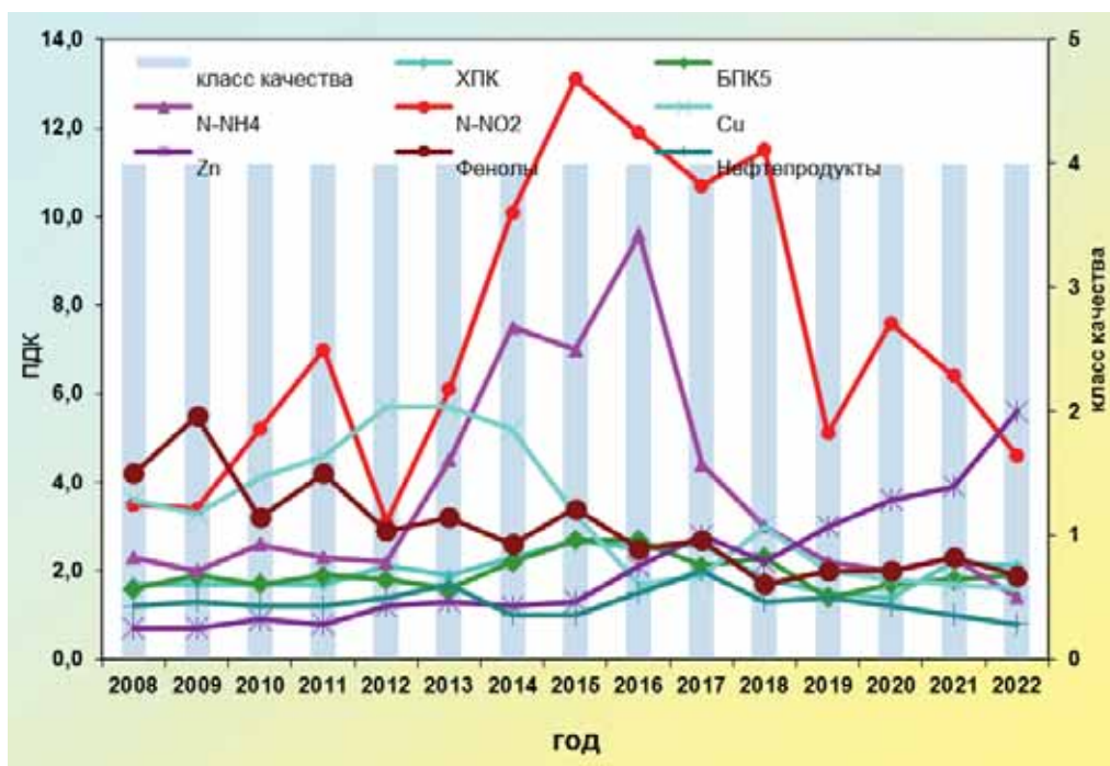
Рис. 3.36. Изменение среднегодовых концентраций отдельных загрязняющих веществ и показателей качества воды р. Ока ниже г. Коломна за многолетний период
